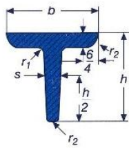
DIN EN 10 055 (T) Größe 30 - 140
