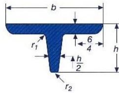
DIN 1024 (TB) Größe 30/60 - 60/120
